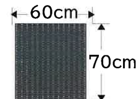
火葬炉間口図
